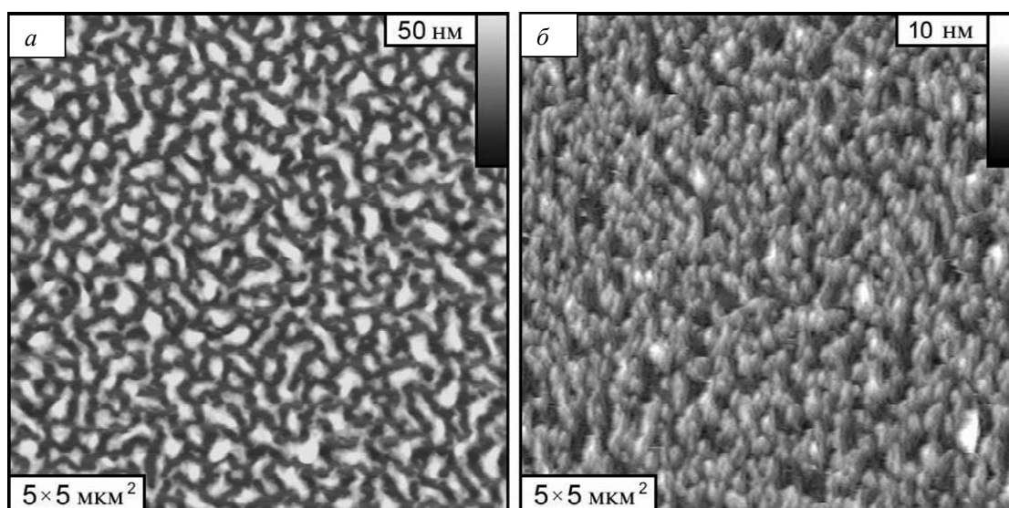
Рис. 2. АСМ-изображения пленки Teflon AF, сформированной на поверхности слюды.
