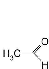
I (ацетальдегид)
