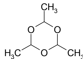
III (паральдегид)
