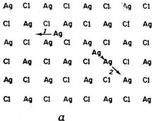
Рис. 13.6. Миграция междузельного иона \text{Ag}^+ : a — путем прямого перескока из одного междузелья в другое (1) и с вытеснением регулярного иона в междузелье (2); б — возможные направления междузельной миграции иона \text{Ag}^+ в \text{AgCl} .
