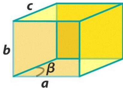
Monoclinic
