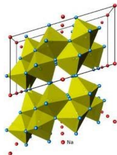
Титанаты, цирконаты
