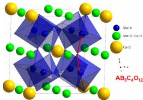
KMS-манганиты
