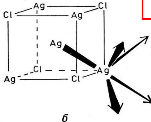
Рис. 13.6. Миграция междузельного иона \text{Ag}^+ : a — путем прямого перескока из одного междузелья в другое (1) и с вытеснением регулярного иона в междузелье (2); б — возможные направления междузельной миграции иона \text{Ag}^+ в \text{AgCl} .
