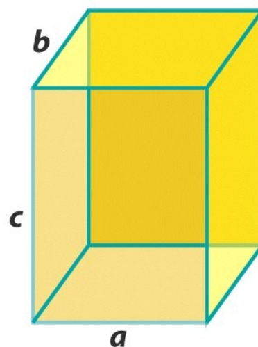
Orthorhombic
