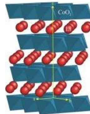
Кобальтиты
